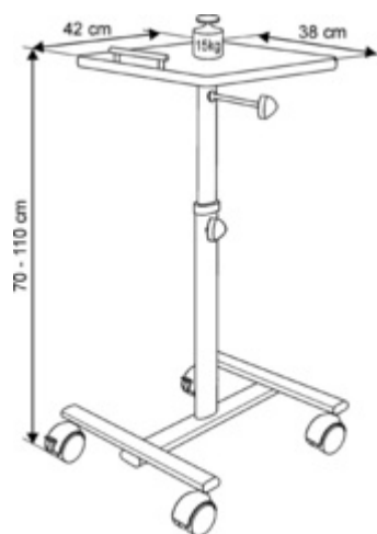
Projektionswagen EuroLine DVP I, Skizze
